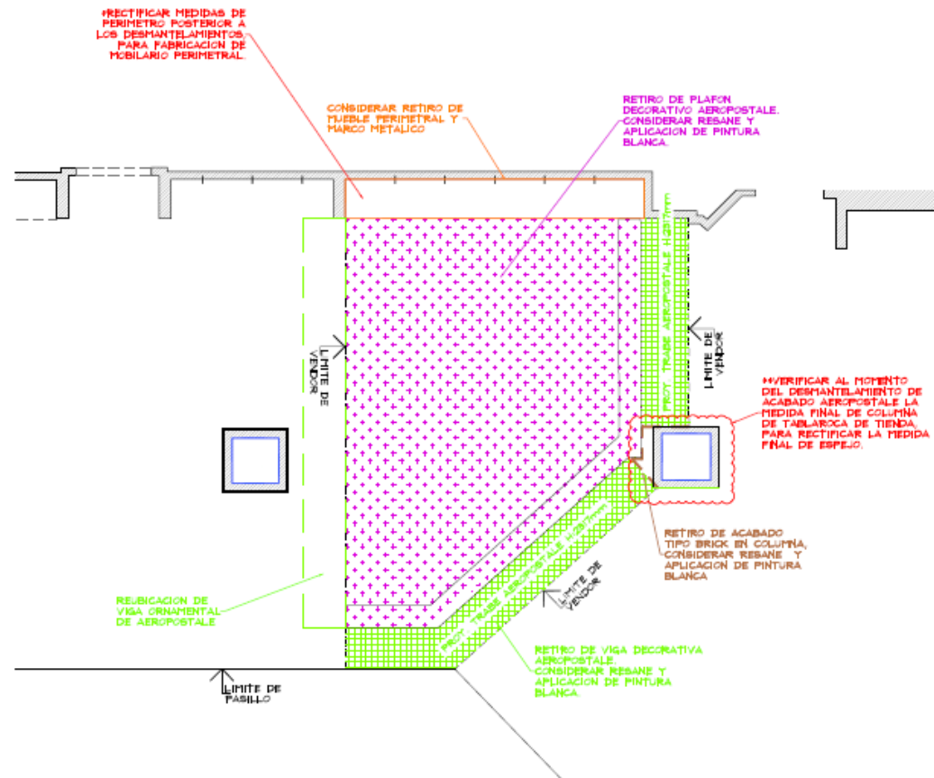
PLANTA DEMOLICIONES ESC. 1:50
