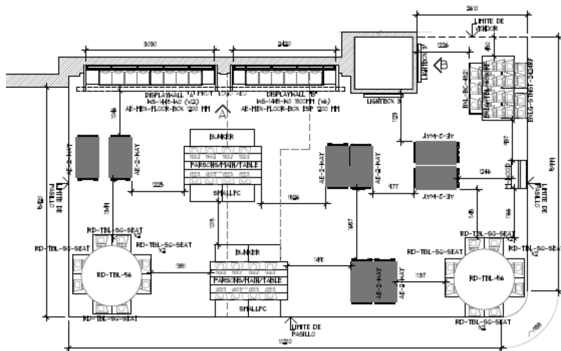
PLANTA ARQUITECTONICA ESC. 1:50
