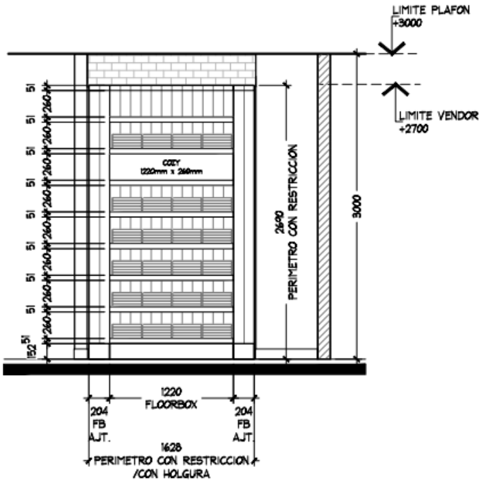
ALZADO B ESC. 1:50
