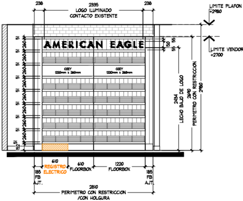
ALZADO A ESC. 1:50
