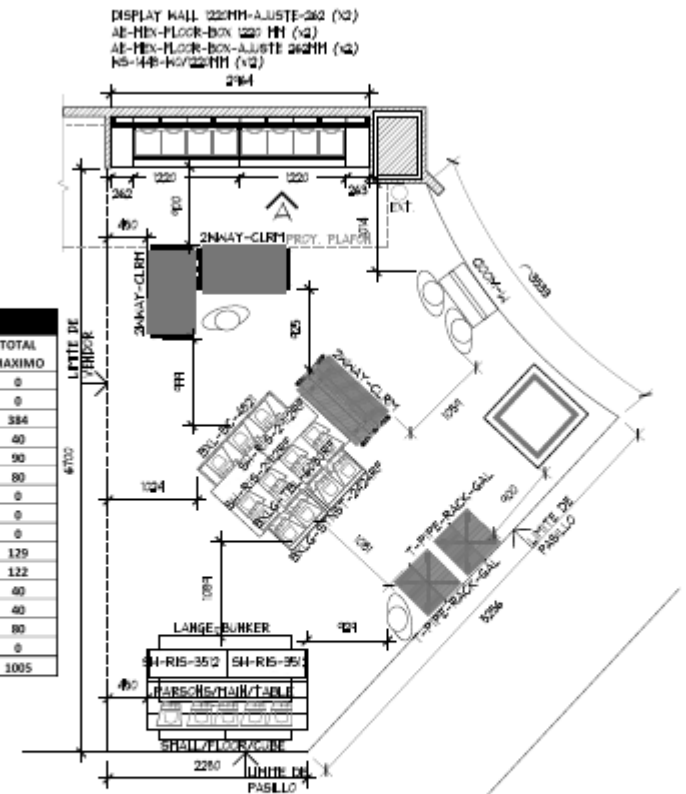
PLANTA ARQUITECTONICA ESC. 1:50
