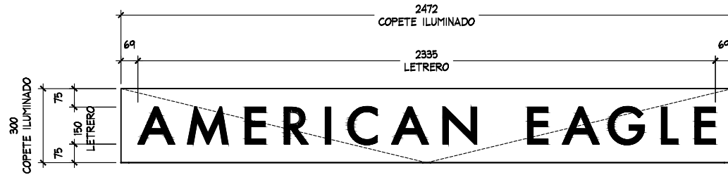
DETALLE LOGO ESC. 1:20
