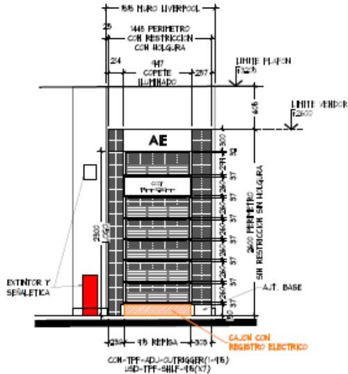
ALZADO C ESC. 1:50
