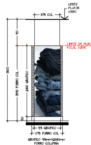
ALZADO F ESC. 1:50
