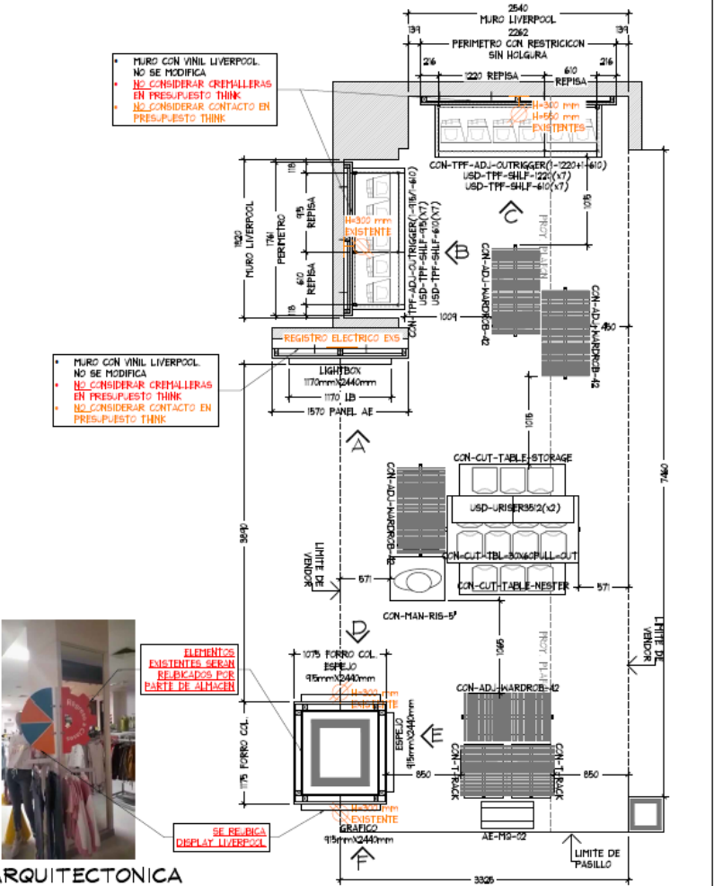
PLANTA ARQUITECTONICA ESC. 1:50
