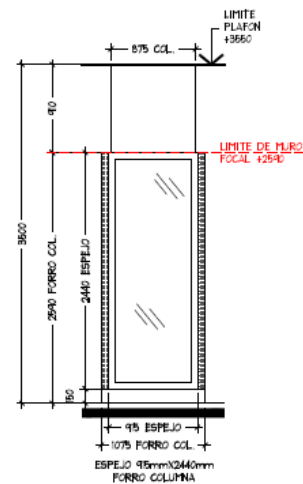
ALZADO D ESC. 1:50
