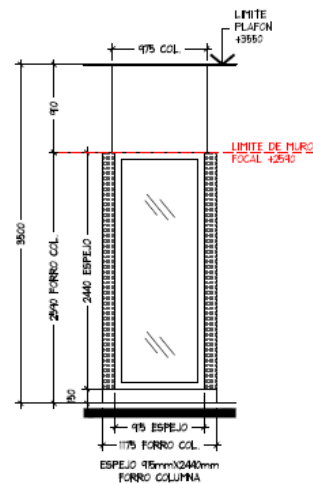
ALZADO E ESC. 1:50
