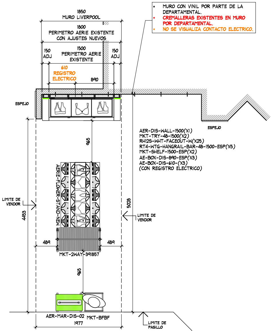
PLANTA ARQUITECTONICA ESC. 1:50
