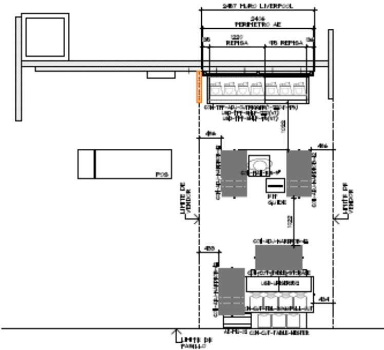
PLANTA ARQUITECTONICA ESC. 1:50
