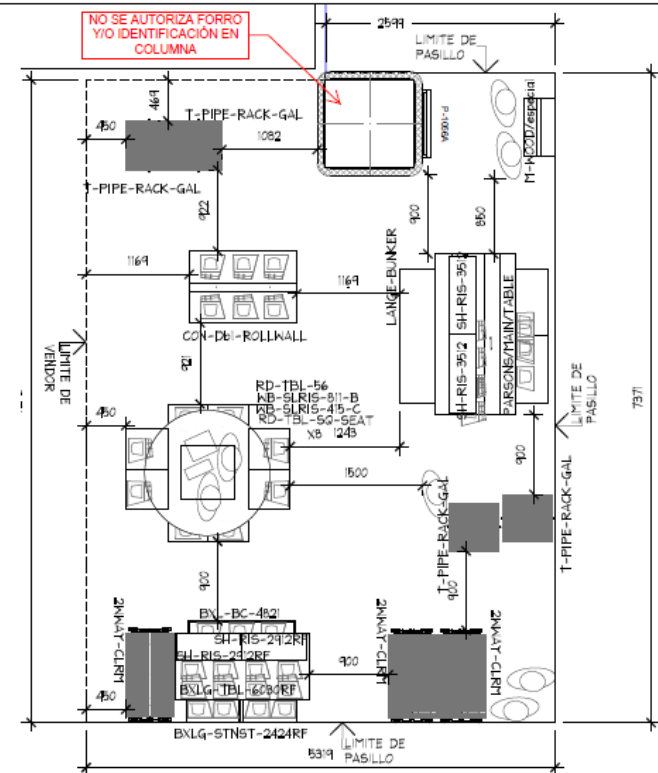
PLANTA ARQUITECTONICA ESC. 1:50
