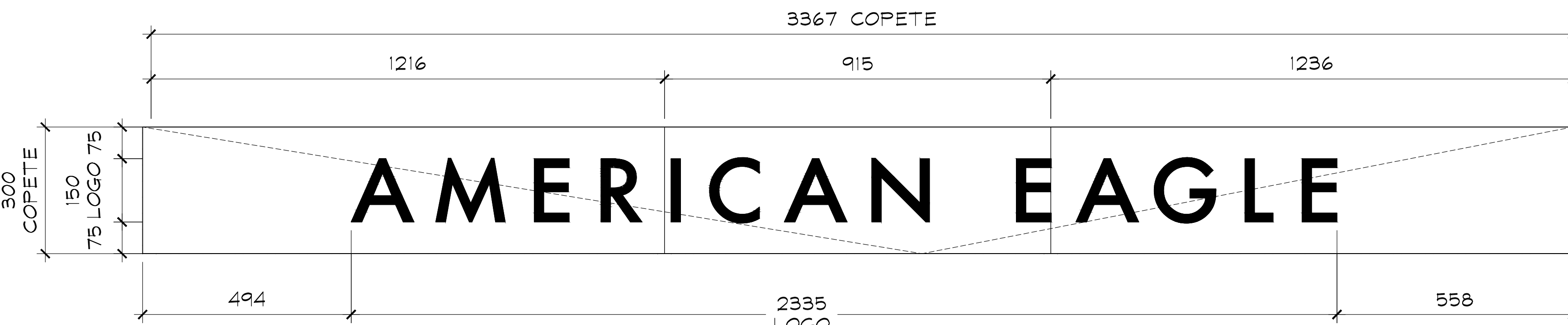
DETALLE LETRERO ESC. 1:20
