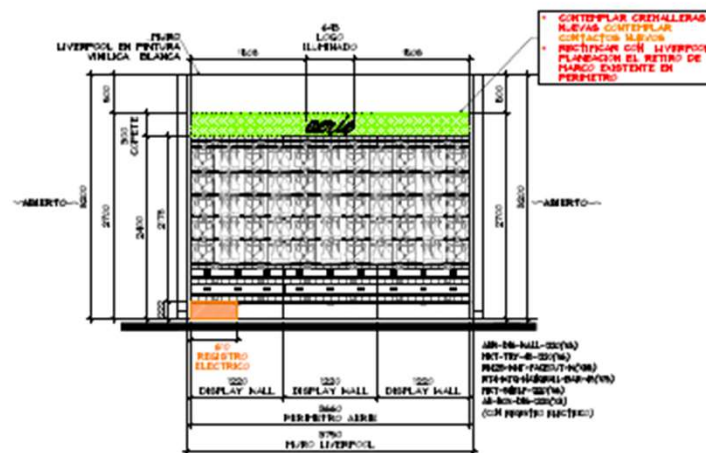
ALZADO A ESC. 1.50
