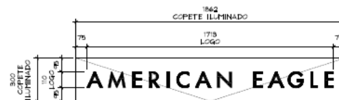
DETALLE LOGO 1-2 ESC. 1:20
