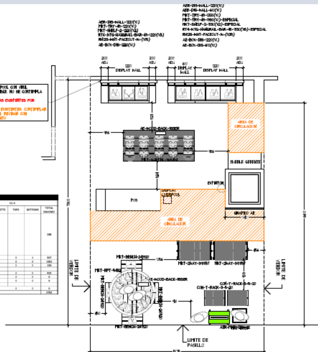
PLANTA ARQUITECTONICA EBC. 1:50
