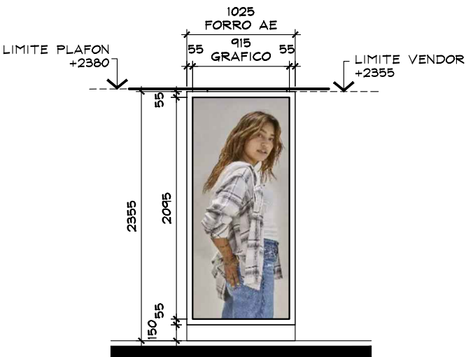
ALZADO E ESC. 1:50
