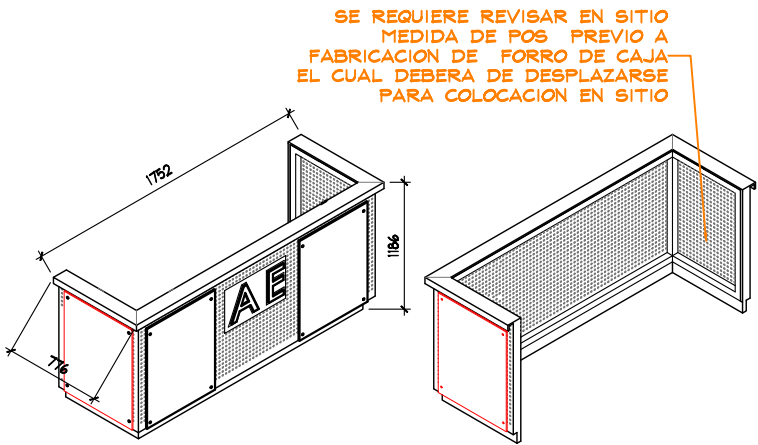
ISOMETRICO TIPO DE FORRO D/CAJA S/E
