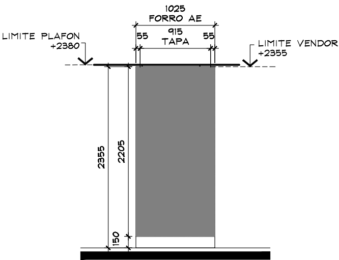
ALZADO G ESC. 1:50
