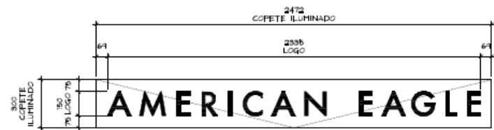
DETALLE DE LETRERO ESC. 1:20
