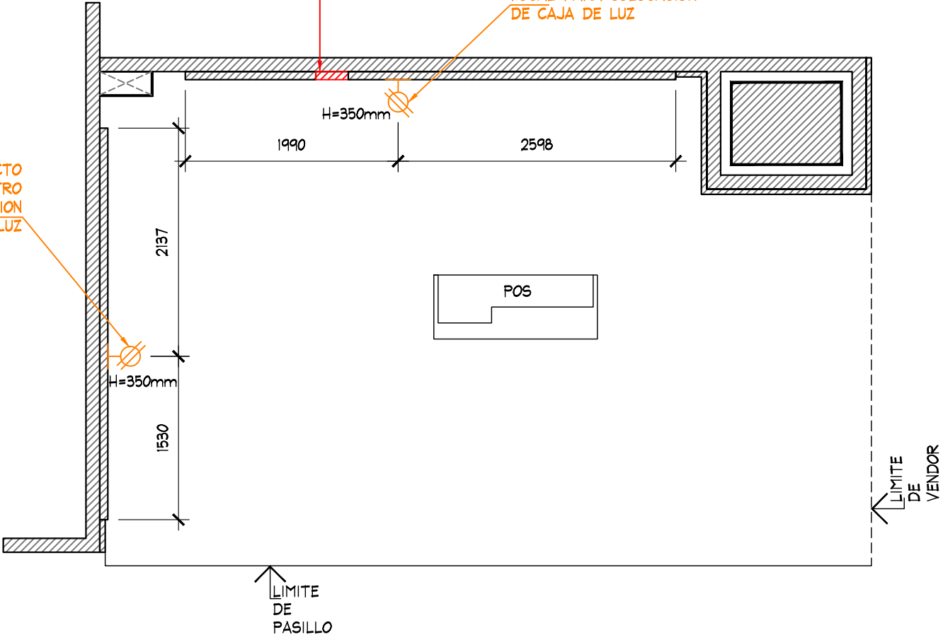
PLANTA DE FUERZA ESC. 1:50
