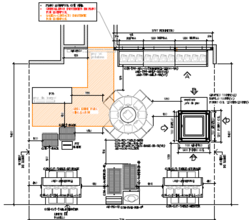
PLANTA ARQUITECTONICA ESC. 1:50
