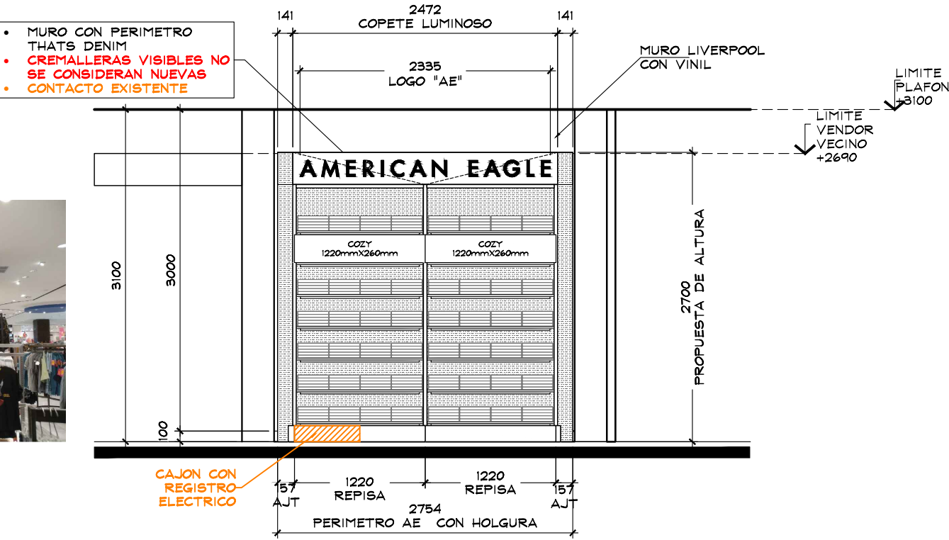
ALZADO A ESC. 1:50
