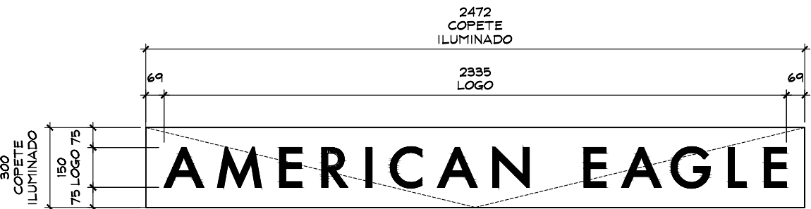
DETALLE LOGO ESC. 1:20
