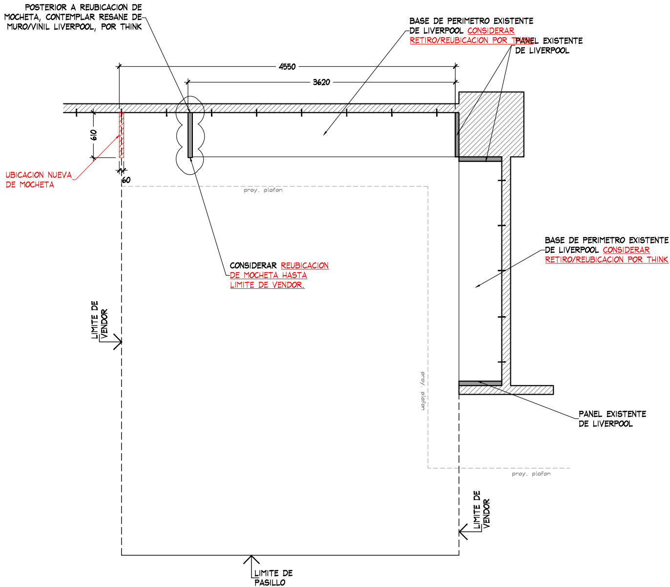
PLANTA DE ADECUACIONES ESC. 1:50
