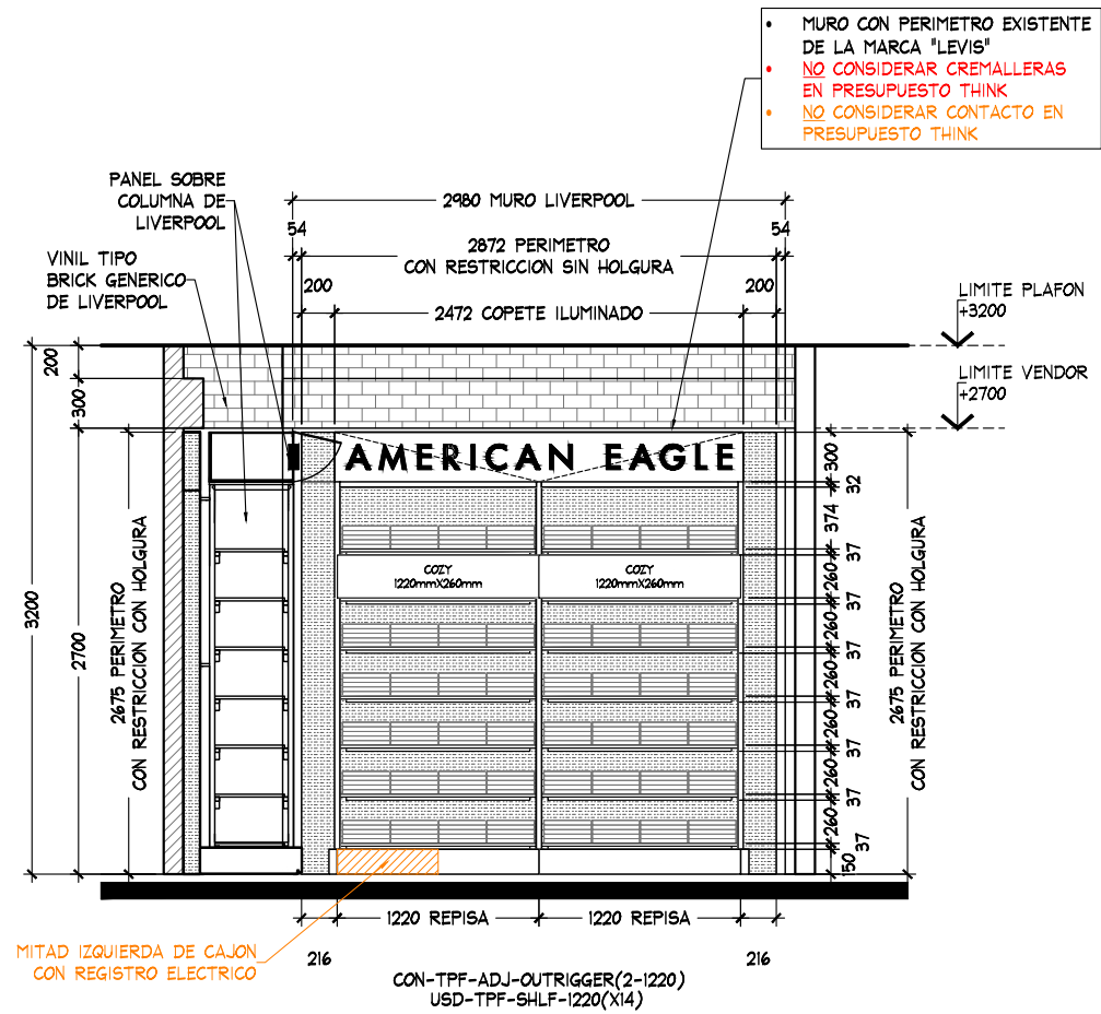
ALZADO B ESC. 1:50
