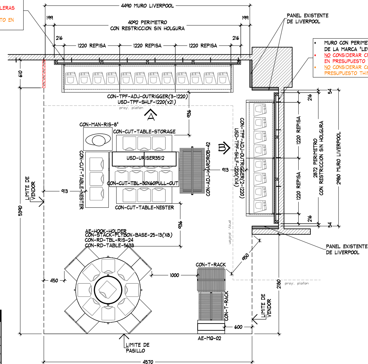
PLANTA ARQUITECTONICA ESC. 1:50
