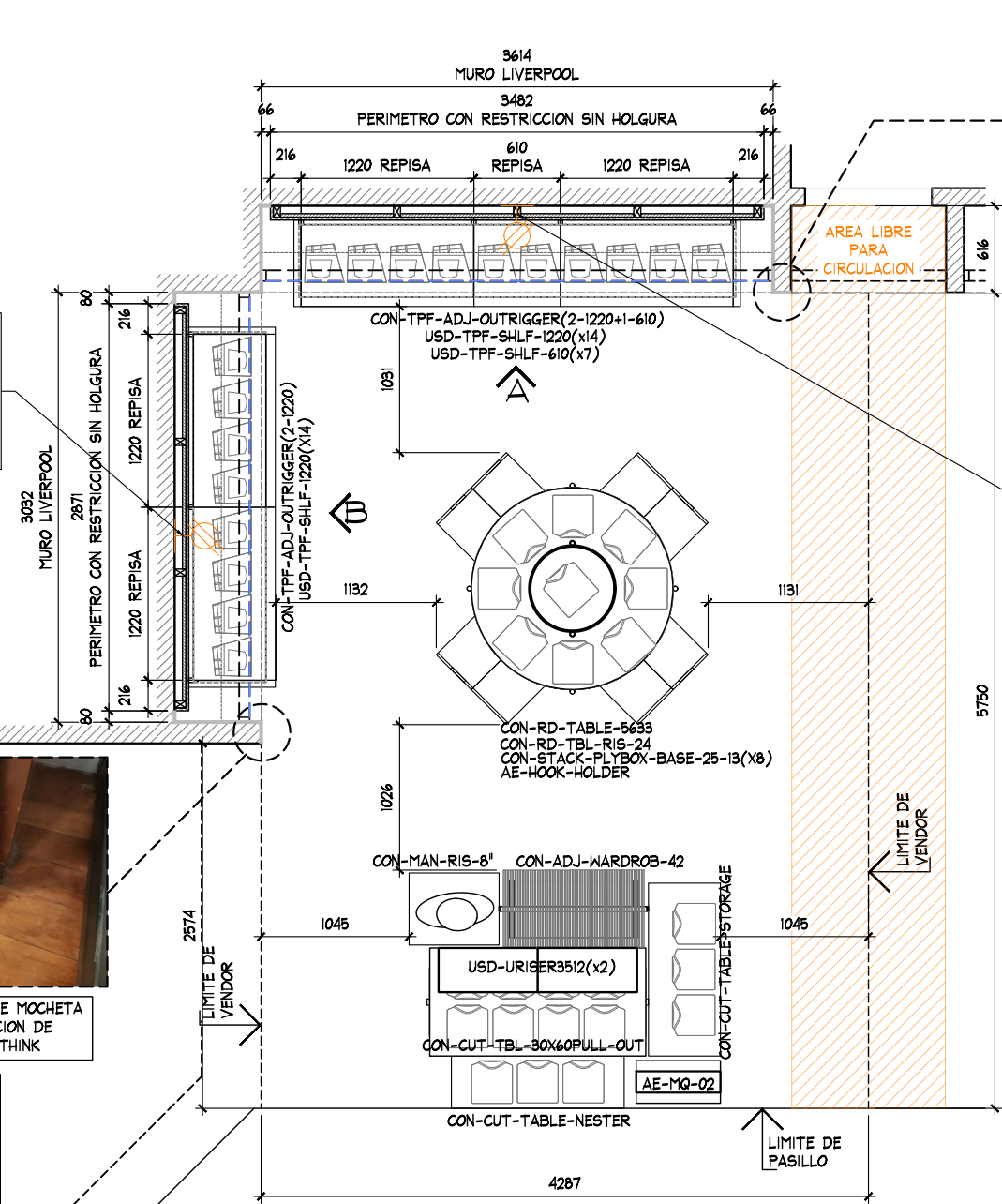
PLANTA ARQUITECTONICA ESC. 1:50
