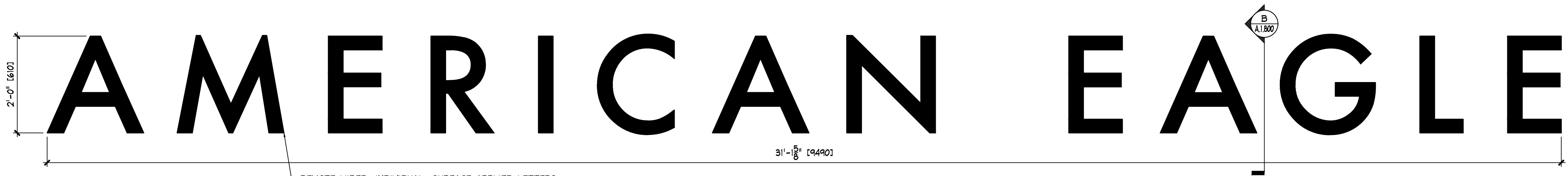
A STOREFRONT SIGN DETAIL A.1.800 SCALE: 1 1/2" = 1'-0" [1:6] (03-21-2016)
