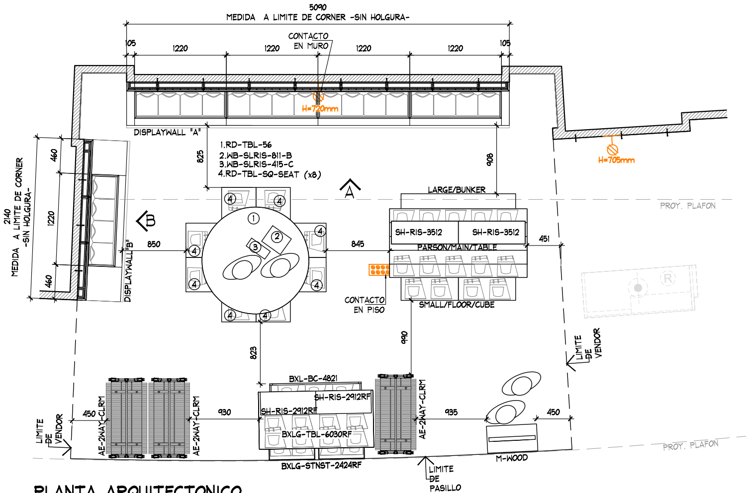
PLANTA ARQUITECTONICO ESC. 1:50
