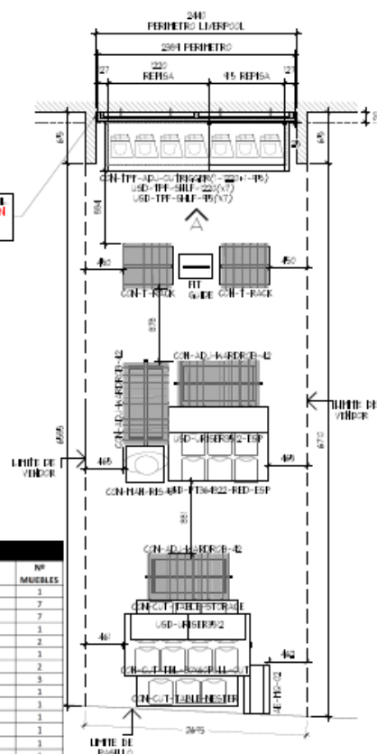
PLANTA ARQUITECTONICA ESC. 1:50
