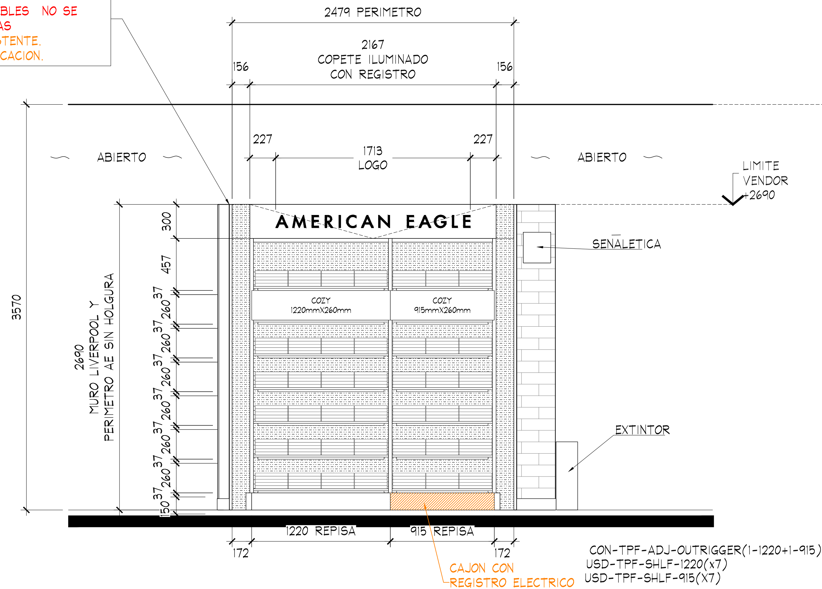
ALZADO A ESC. 1:50
