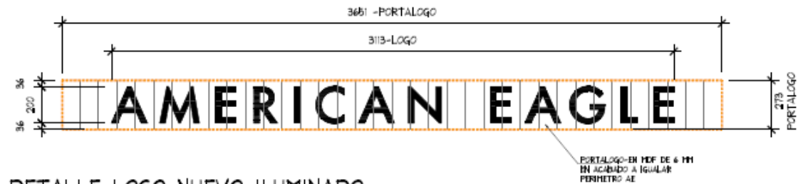
DETALLE LOGO NUEVO ILUMINADO ESC. 1:20
