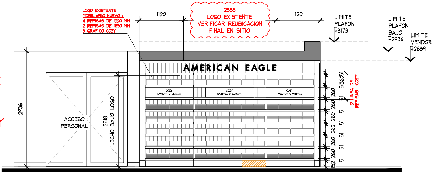
ALZADO A ESC. 1:50
