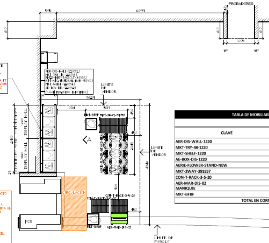
PLANTA DE MOBILIARIO ESC. 1:50
