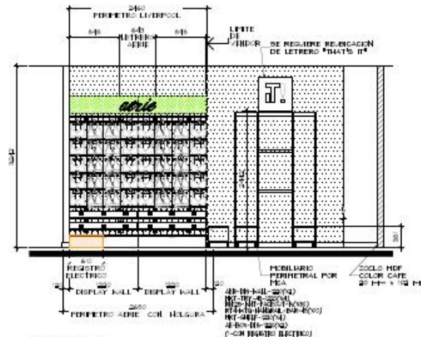
ALZADO A ESC. 1:50
