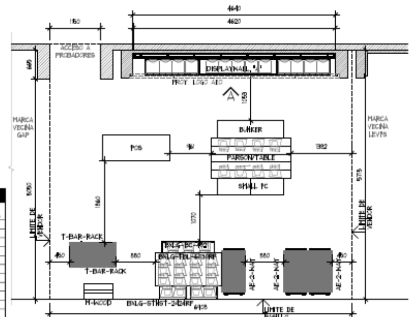
PLANTA ARQUITECTONICA ESC. 1:50
