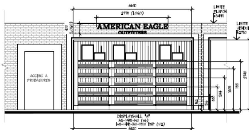
ALZADO A ESC. 1:50
