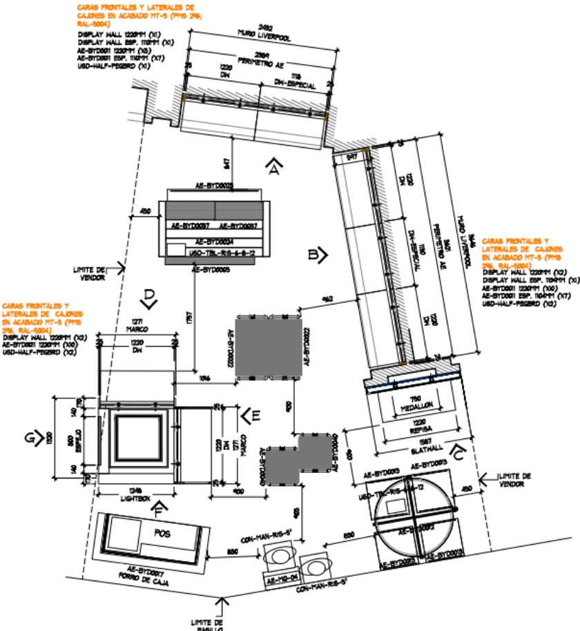
PLANTA DE MOBILIARIO ESC. 1:50
