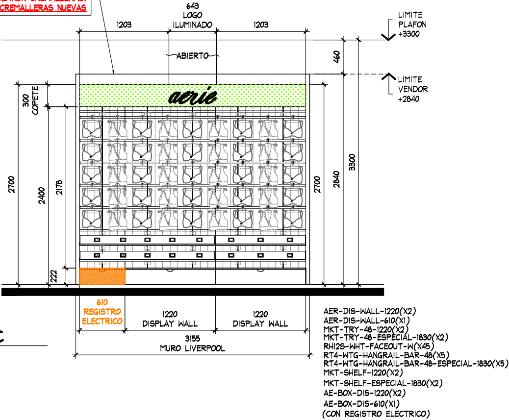
ALZADO C ESC. 1:50
