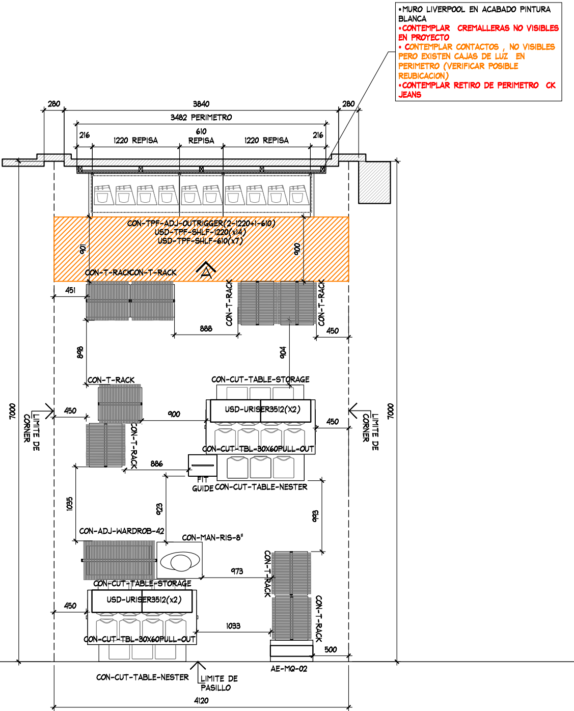
PLANTA PROYECTO ESC. 1:50
