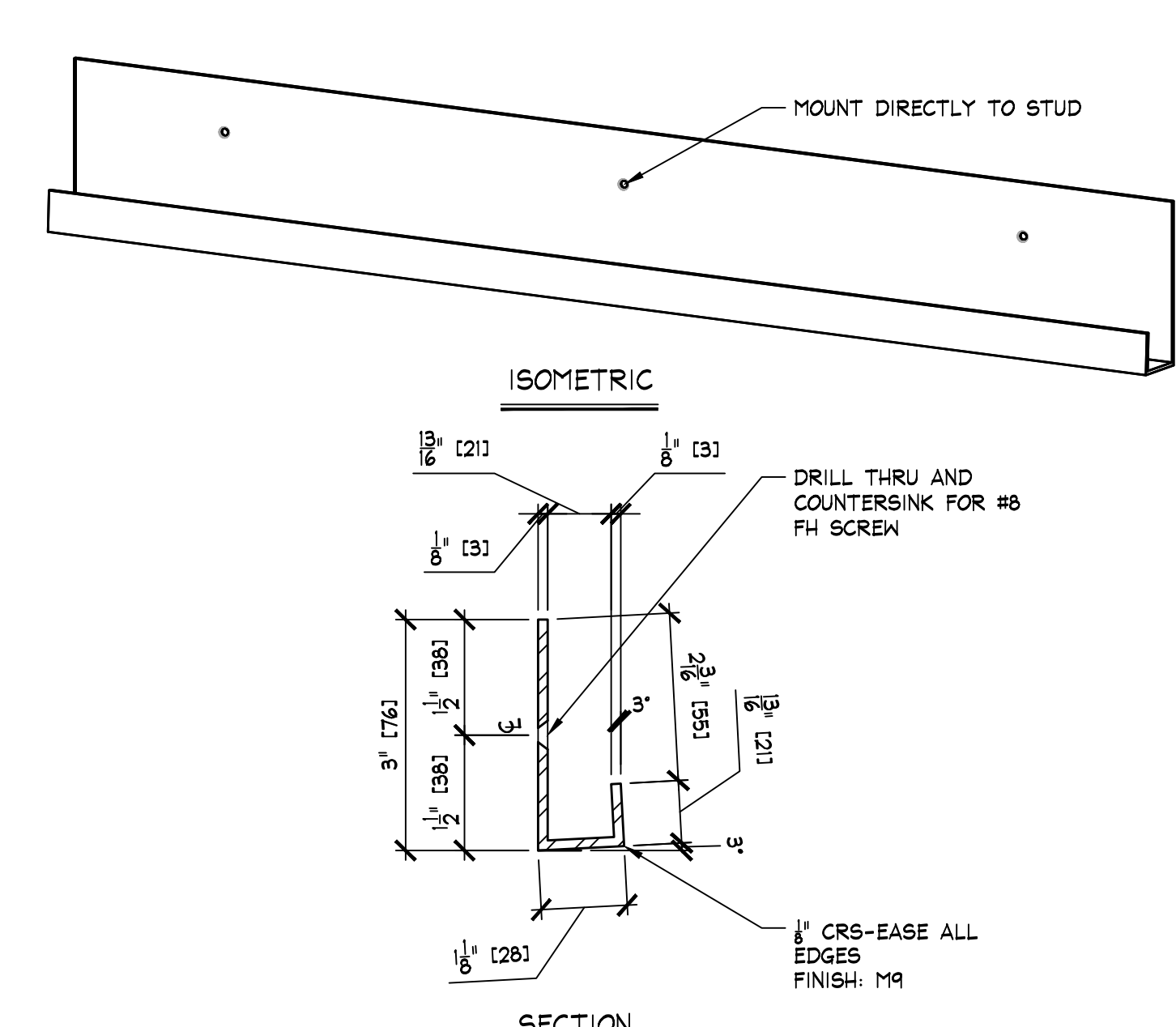
H MIRROR WALL BRACKET SCALE: 6" = 1'-0" [1:2]
