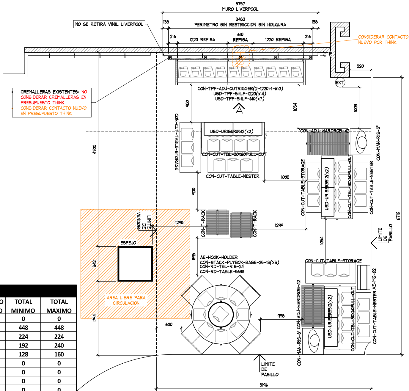
PLANTA ARQUITECTONICA ESC. 1:50
