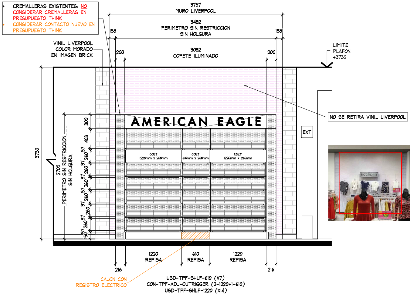
ALZADO A ESC. 1:50
