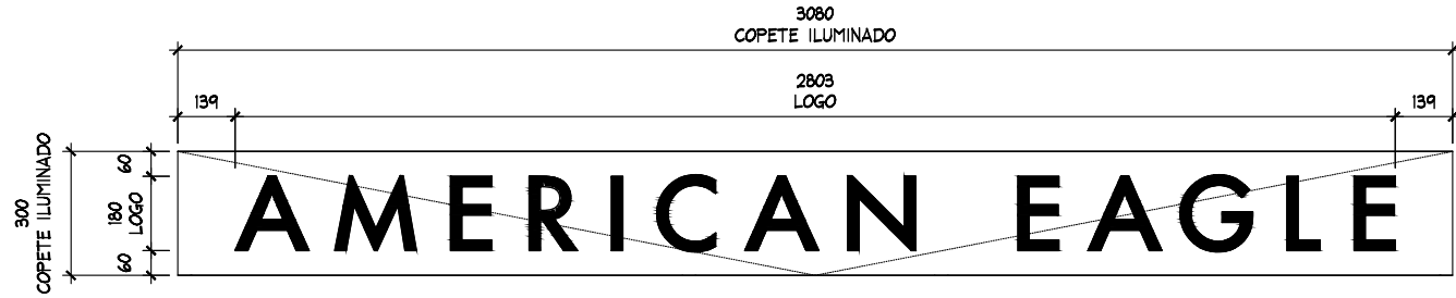
DETALLE LOGO ESC. 1:20
