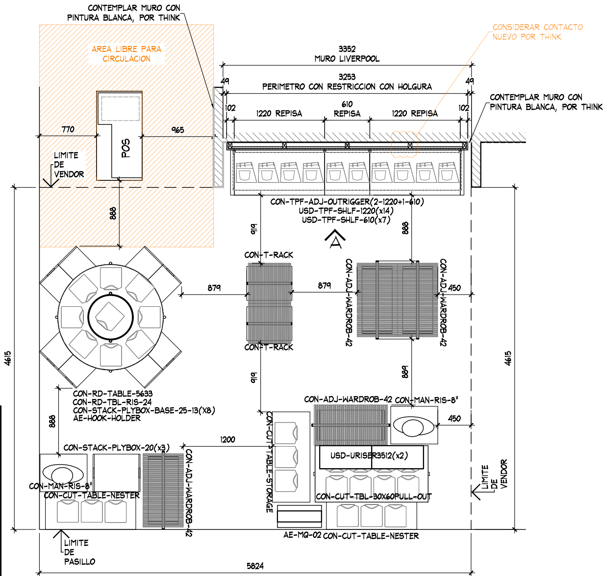
PLANTA ARQUITECTONICA ESC. 1:50
