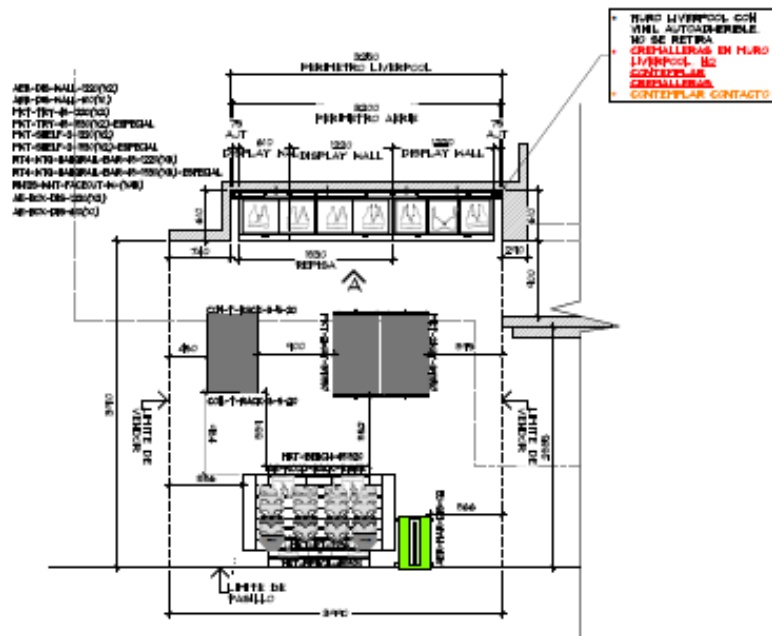
PLANTA GENERAL ESC. 1:50
