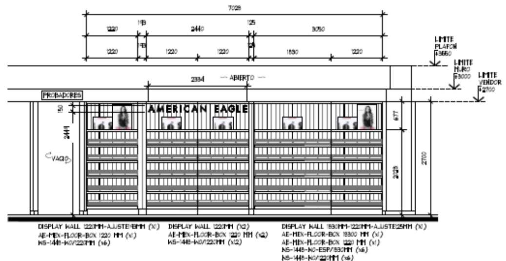
ALZADO A ESC. 1:50
