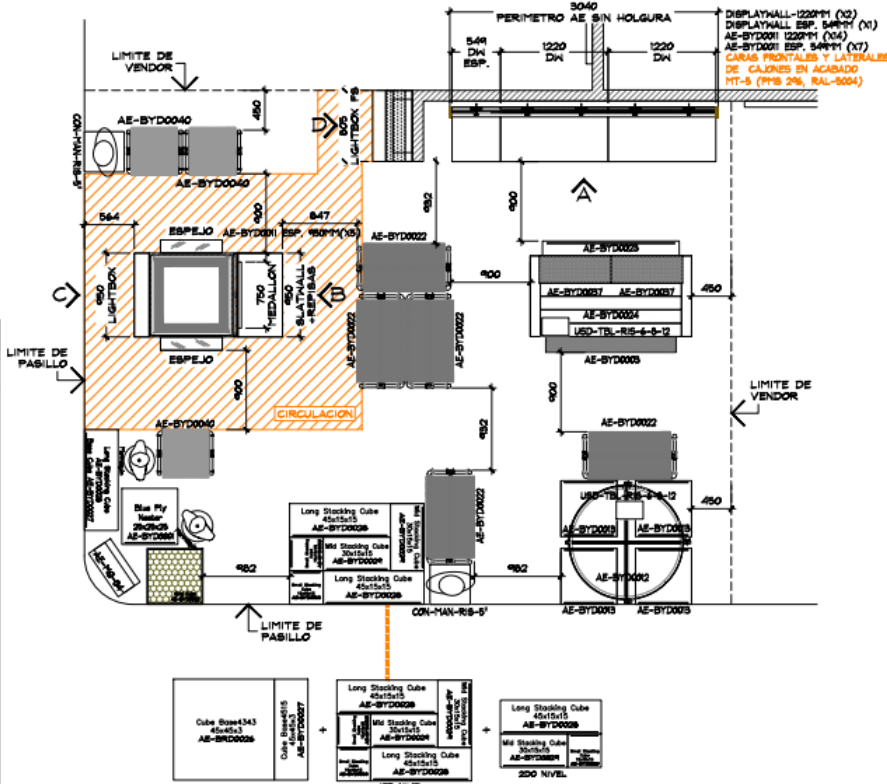
PLANTA MOBILIARIO ESC. 1:50
