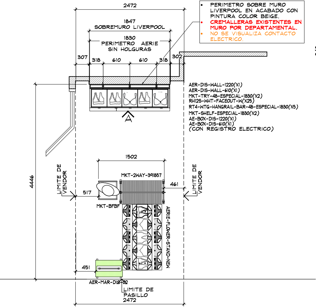
PLANTA ARQUITECTONICA ESC. 1:50
