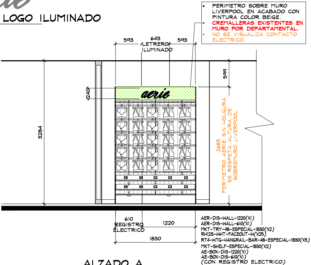
ALZADO A ESC. 1:50
