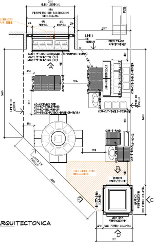
PLANTA MOBILIARIO
