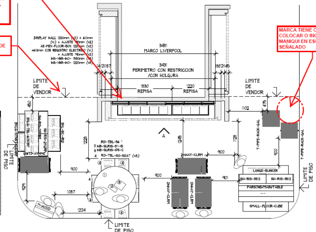
PLANTA MOBILIARIO OP-1 ESC. 1:50
