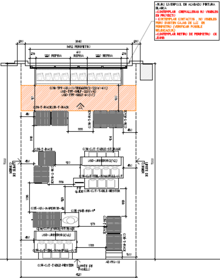
PLANTA PROYECTO ESC. 1:50
