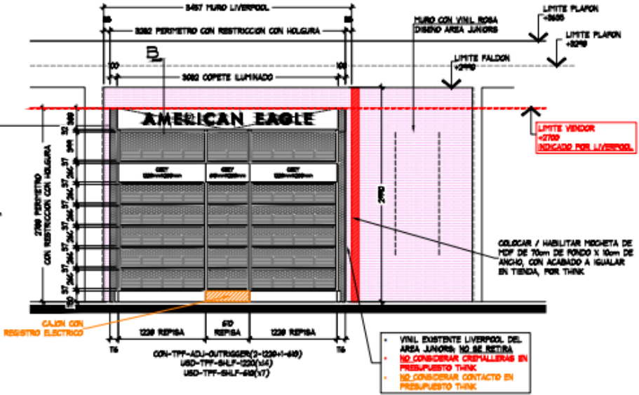
ALZADO A ESC. 1:50
