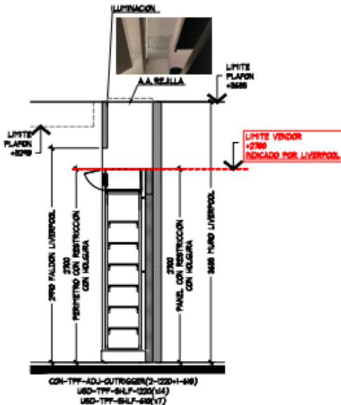
CORTE INDICADA 1:50
