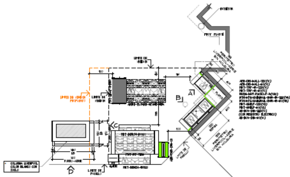
PLANTA ARQUITECTONICA ESC. 1:50
