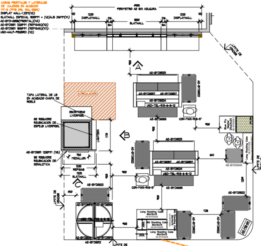
PLANTA GENERAL ESC. 1:50
