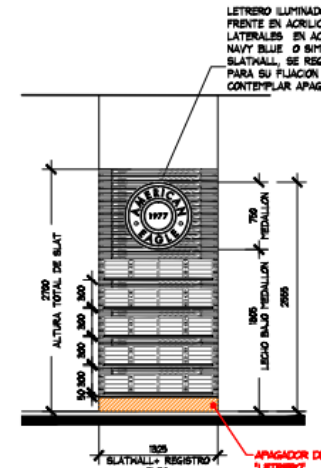
ALZADO C ESC. 1:50
