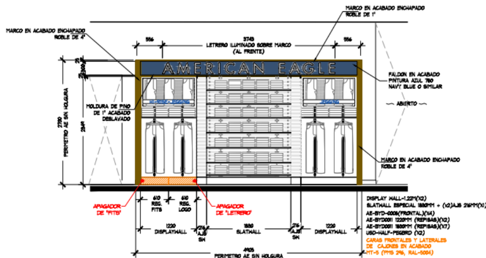
ALZADO A ESC. 1:50
