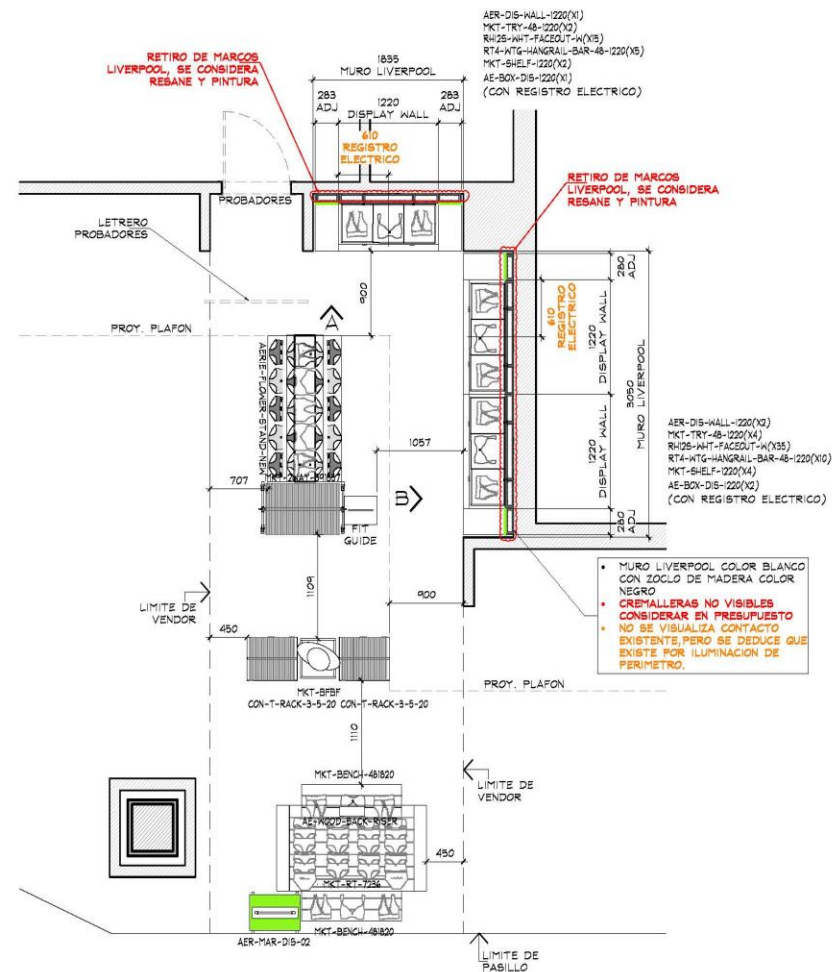
PLANTA ARQUITECTONICA ESC. 1:50
