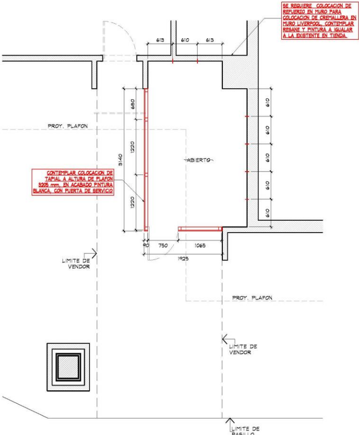
PLANTA CREMALLERAS ESC. 1:50
