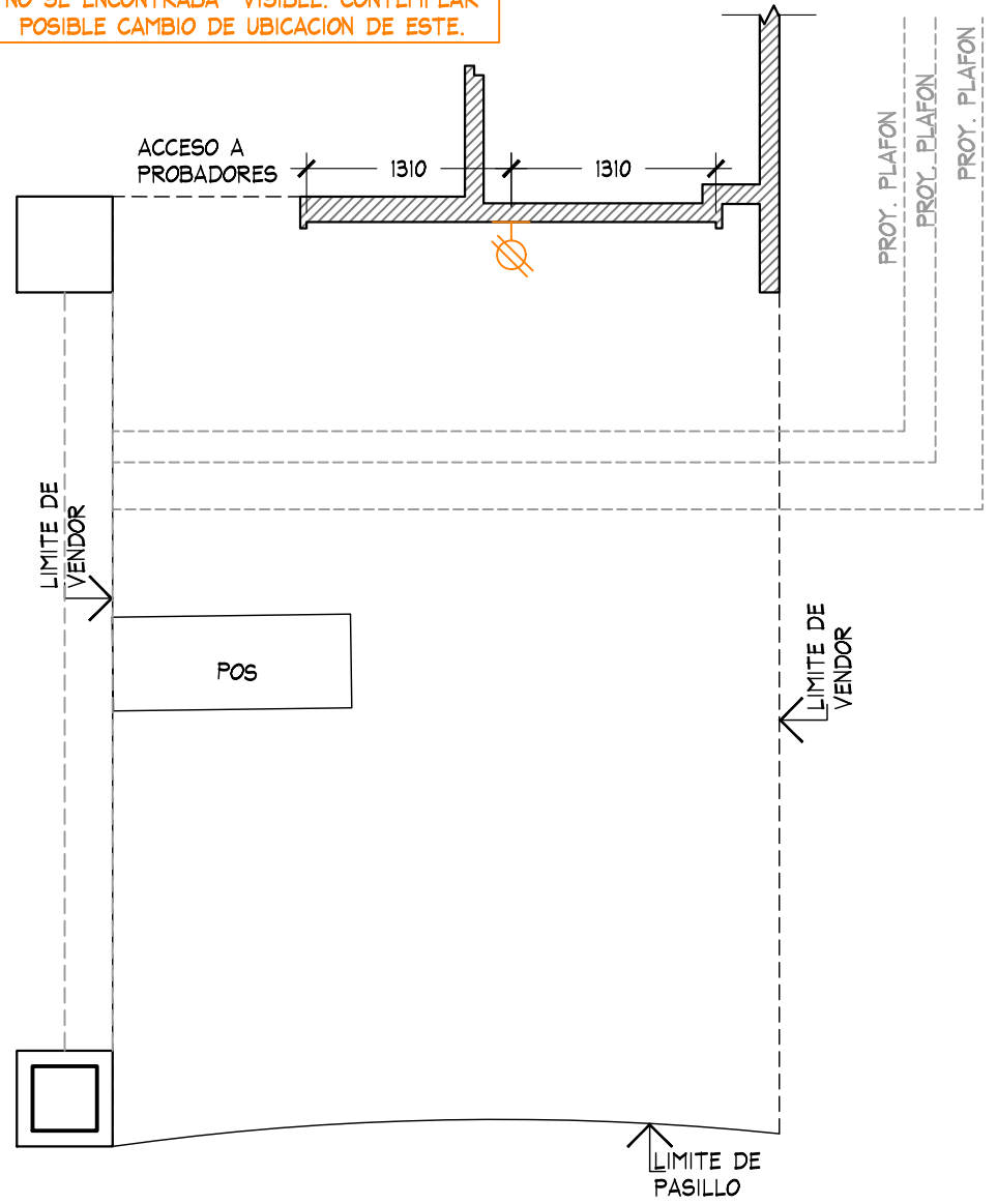
PLANTA DE FUERZA ESC. 1:50
