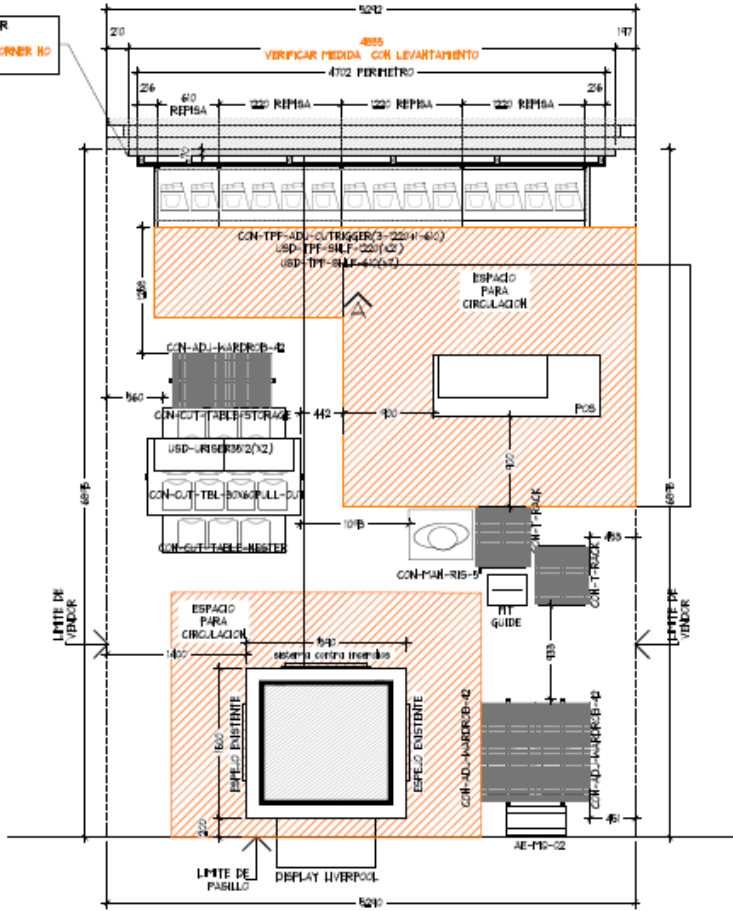
PLANTA ARQUITECTONICA ESC. 1:50
