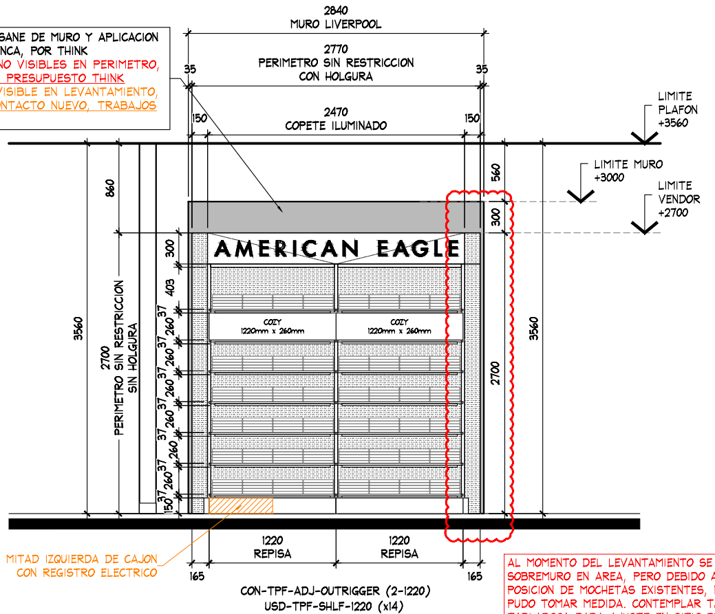
ALZADO B ESC. 1:50
