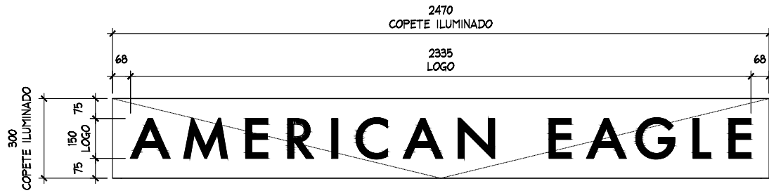
DETALLE LOGO ESC. 1:20
