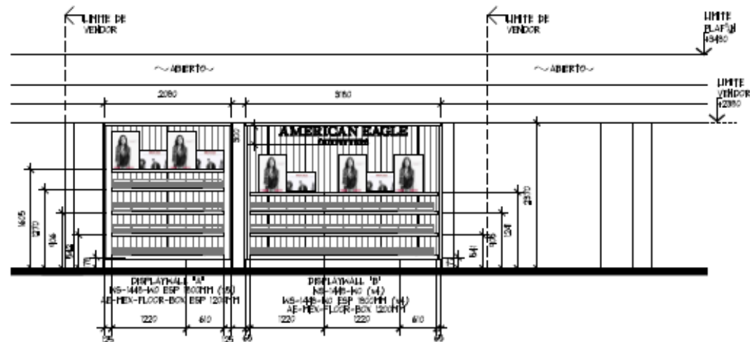
ALZADO A ESC. 1:50
